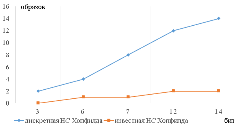
Рисунок 3 – Сравнение информационной емкости известной нейронной сети Хопфилда с предложенной
