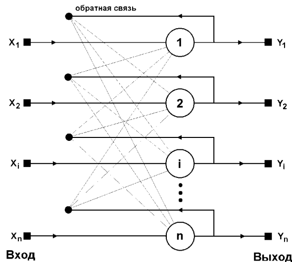
Рисунок 1 – Структура нейронной сети Хопфилда
